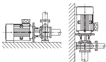
Fig. 5: Widok Atmos GIGA-B
