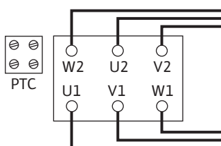
Fig. 16: Collegamento Y- \Delta
