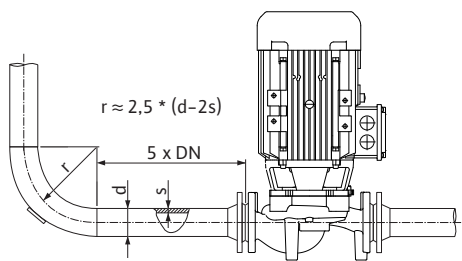
Fig. 13: Tramo de estabilización delante y detrás de la bomba
