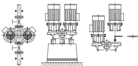
Fig. 4: Vista Wilo-Atmos GIGA-D
