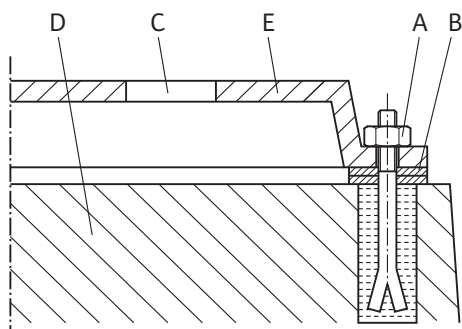
Fig. 12: Przykład połączenia śrubowego z fundamentem
