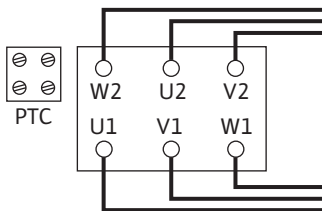
Fig. 16: Conmutación Y- \Delta
