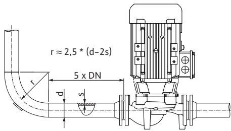
Fig. 13: Percorso di stabilizzazione a monte e a valle della pompa
