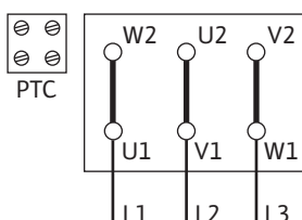
Fig. 14: Collegamento \Delta
