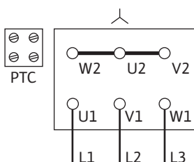
Fig. 15: Collegamento Y
