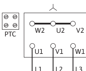
Fig. 15: Połączenie Y
