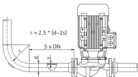
Fig. 13: Odcinek wyrównywania przed i za pompą
