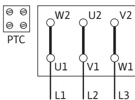
Fig. 14: Połączenie Y-Δ
